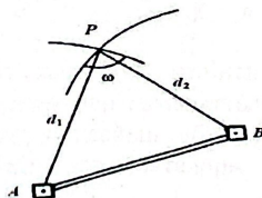
7-сурет – Сызықтық қиылыстыру әдісі
