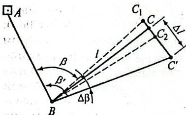
11-сурет - Жобалық бұрышты жер бетінде құрудың сұлбасы
