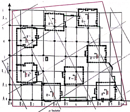
3-сурет - Тұрғын үй кешенінің құрылыс торы
