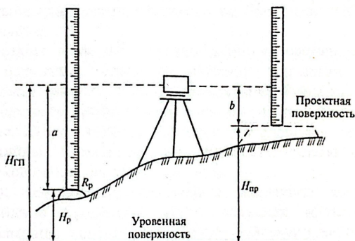
13-сурет - Жобалық белгіні жер бетіне көшіру сұлбасы
