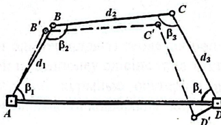
9-сурет – Қатар және қатар-сызықтар әдісі
