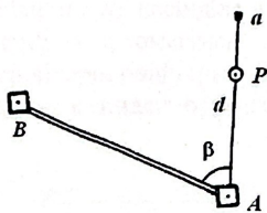
8-сурет – Полярлық координаталар әдісі
